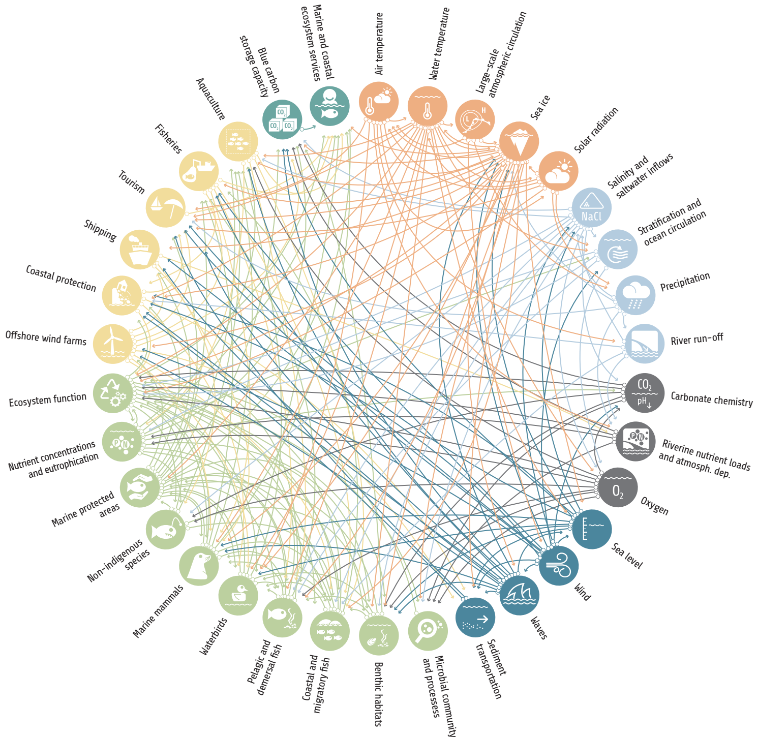
Abbildung 2. Verbindungen zwischen den in diesem Faktenblatt genutzten Parametern.
